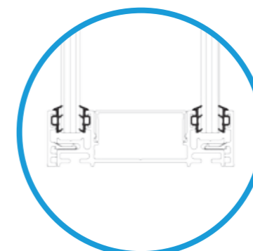
Onderprofiel ClearVision 100
