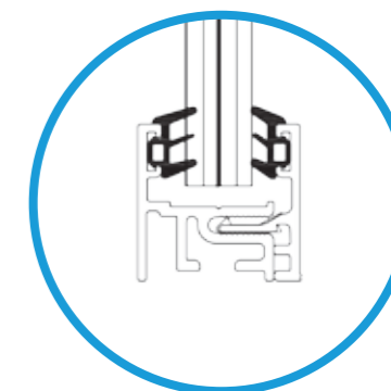
Onderprofiel ClearVision 25 en 30
