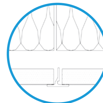
Moduulovergang T100
