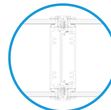
Moduulovergang T100 open
