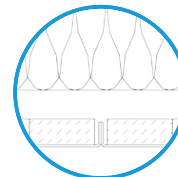
Moduulovergang V100
